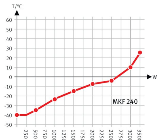
Диаграмма компенсации тепла
