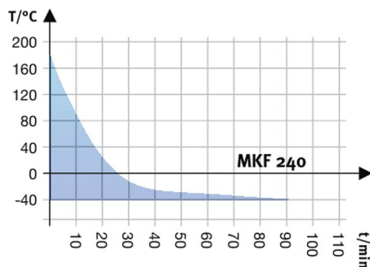
Кривая охлаждения
